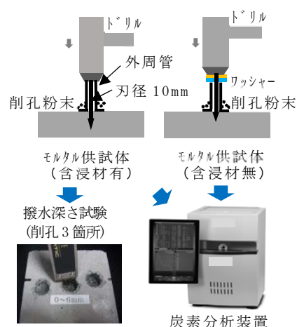
Fig. 1 試験方法
